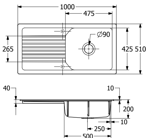
Abb. zeigt Chromite.
