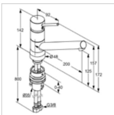
Unterfenstermontage
