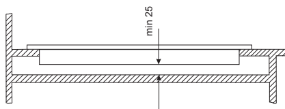
Einbau in der Arbeitsplatte des tragenden Schanks.
