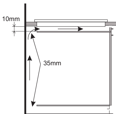
Einbau in der Arbeitsplatte des tragenden Schanks.
