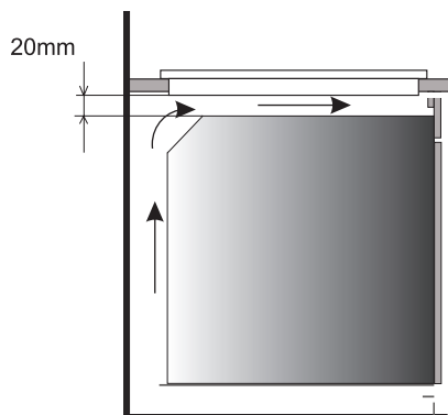
Aménagement dans le plateau de travail au-dessus d'un four avec ventilation.
